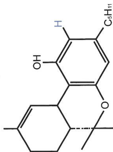
delta 9-THC
